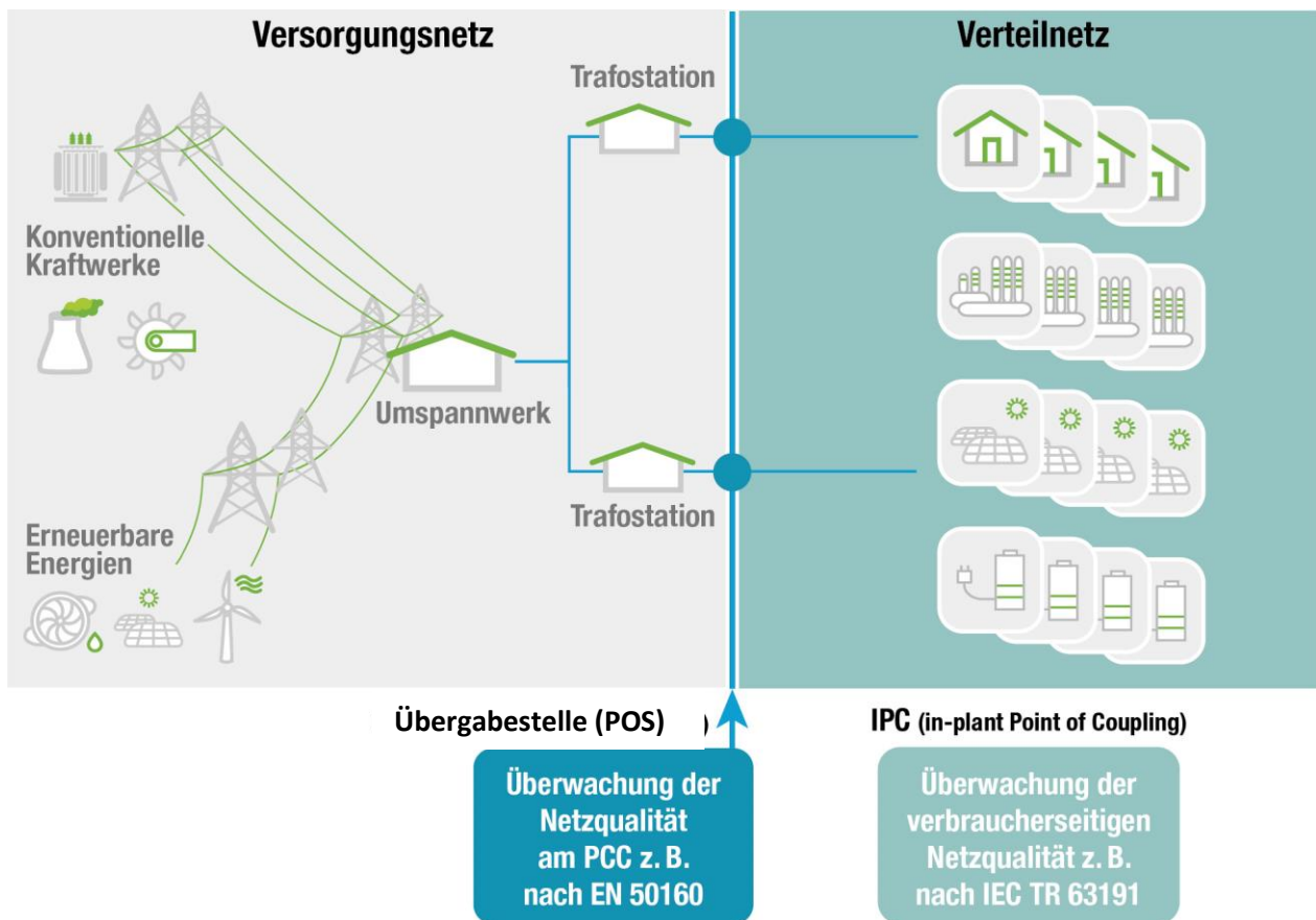
Bild 7: Überwachung der Netzqualität am POS und IPC (vereinfachte Darstellung)
